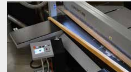
Überlanges (6 m ) Massivholz sägen
