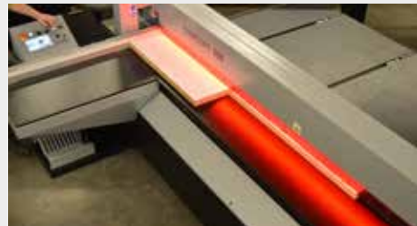
Statusanzeige rot: Achtung, Druckbalken senkt sich
